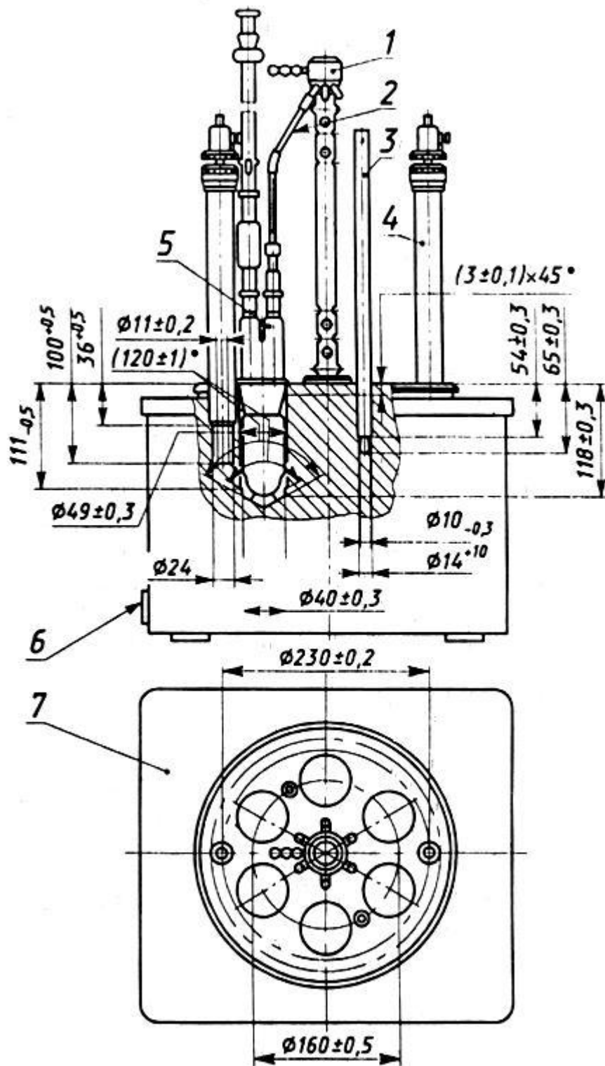
1 - распределитель; 2 - капилляр; 3 - контрольный термометр; 4 - контактный термометр; 5 - испытательный сосуд; 6 - клемма; 7 - алюминиевый блок Черт.1
